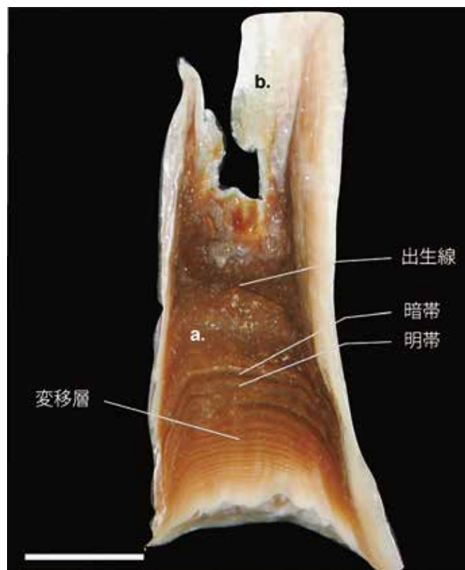
図 1. ミンククジラ耳垢栓切片 a : コア (成長層が形成される), b : アウターカバリング, スケールバー : 5 mm
