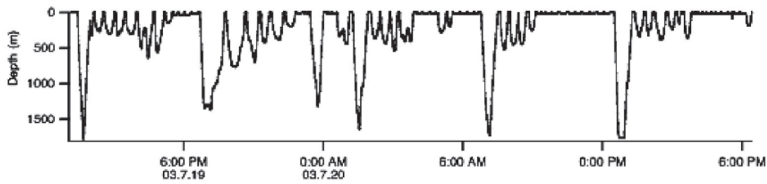
図5 2003年に房総沖で得られたツチクジラの潜水深度時系列データ
