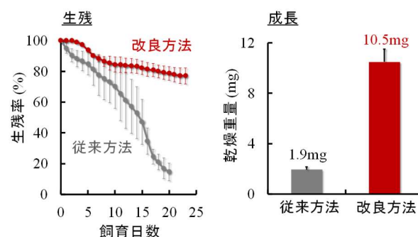
図 2. 従来方法と改良方法 (水流飼育装置+ガザミゾエア幼生給餌) で飼育したマダコの生残率の推移 (左) とふ化後 20 日の乾燥重量 (右)
