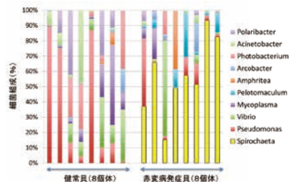
アコヤガイ健康貝と赤変病発症貝における細菌組成。検出率の高い順に上位10属を表示。スピロヘータ（黄色）は病貝に特異的かつ普遍的に存在した。
