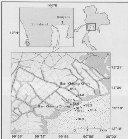
図1. Samut Songkhram県Khlong Khon地区における調査地点。St.5は自然林、St.6とSt.7は植林地にある。図中白抜きの部分は粗放のエビ養殖場。現在のマングローブ縁辺は破線で示した付近（地図は1991年測量に基づき作成されている）。
