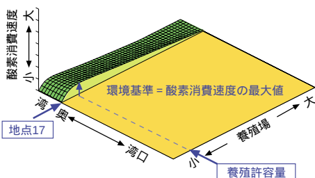
図2c：環境基準で求めるべき 酸素消費速度の最大値（地点17）
