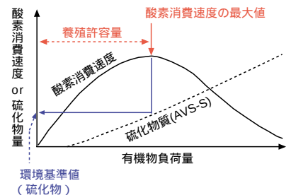
図1：底質の酸素消費速度に基づく 環境基準（硫化物）の模式図
