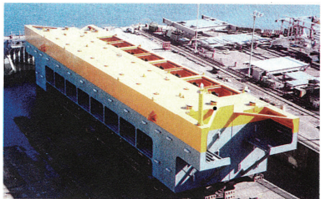
下波・蔭淵地区沖合養殖場造成工事（多機能浮消波堤）
