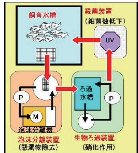
図1 閉鎖循環飼育の模式図
