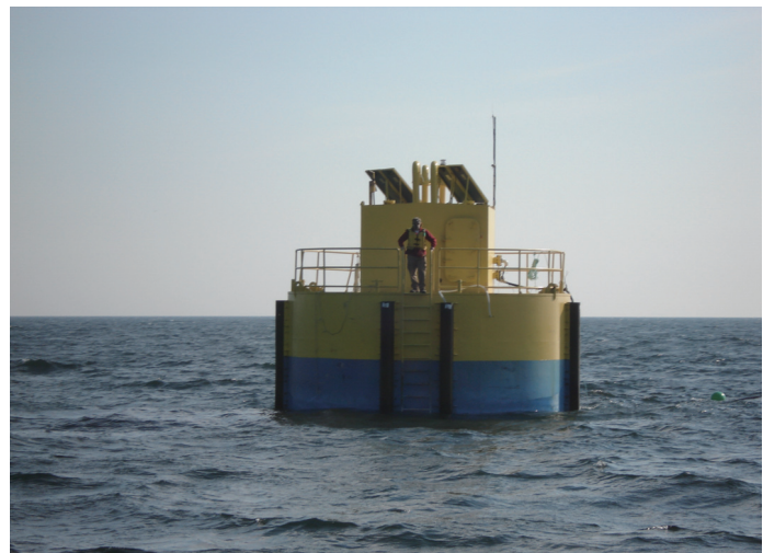
写真2 沖合養殖イケス用自動給餌ブイ (ニューハンプシャー州)
