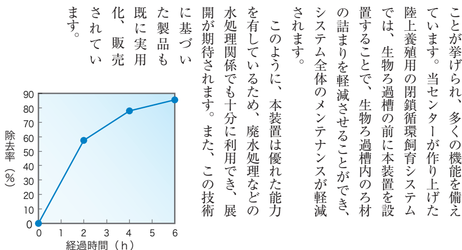
図3. 泡沫分離処理による植物プランクトンの除去率。
