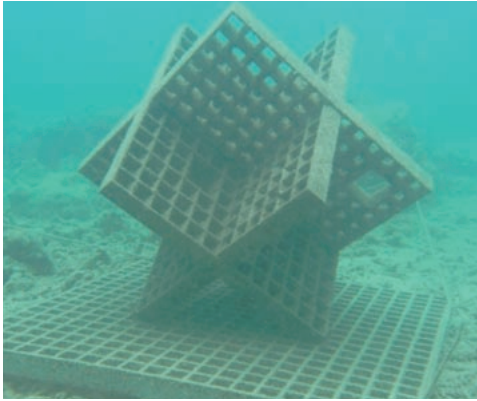
写真1. 4枚の格子状パネルを組み合わせたサンゴ増殖用構造物。
