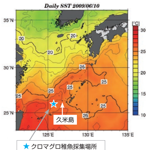
図. クロマグロ稚魚の採集位置と表面水温。
