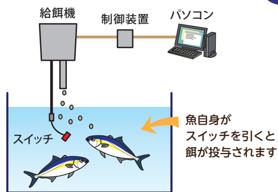
図1. 自発摂餌を利用した自動給餌システム概念図
