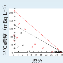
図2 懸濁態 137 Csと塩分の関係
