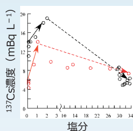
図1 溶存態 137 Csと塩分の関係
