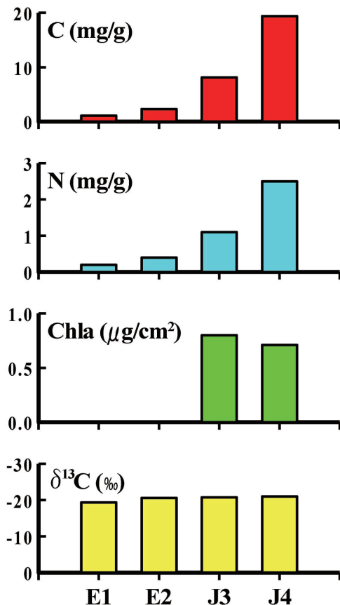
図3 東シナ海北部と日本海西部の堆積有機物組成の比較 東シナ海五島列島沖 (E1:250m, E2:400m), 日本海日御碕沖 (J3:200m, J4:300m); C: 有機炭素量, N: 有機窒素量, Chla: 植物色素量, \delta^{13}\text{C} : 有機炭素安定同位体比。
