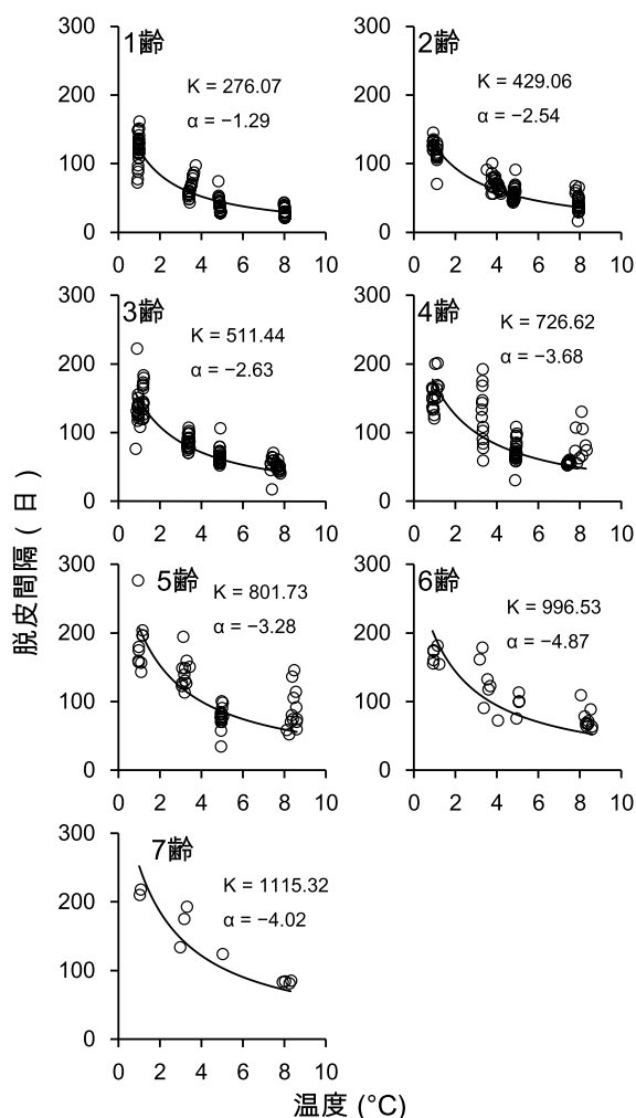
図3. ズワイガニ稚ガニの飼育温度と脱皮間隔の関係 K と \alpha は有効積算温度法則の式の熱定数と発育臨界点。
