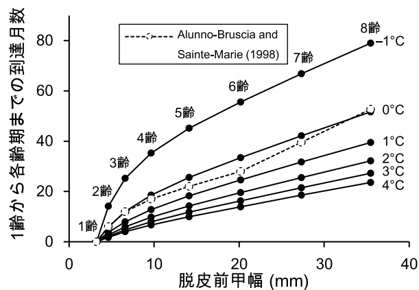
図5. ズワイガニ稚ガニの脱皮前甲幅と、 -1 \sim 4^{\circ}\text{C} 下における1 齢から各齢期までの推定到達月数の関係 白丸はカナダ大西洋岸のセントローレンス湾北西部で推定されている月数。
