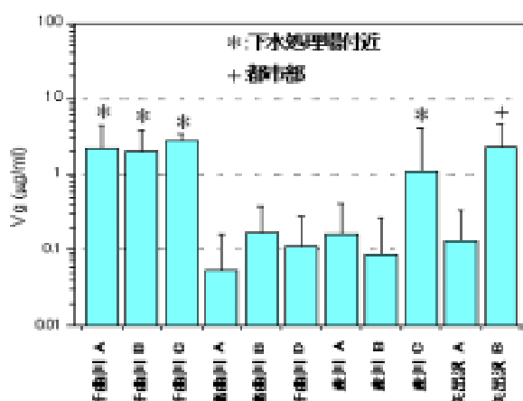
図2 河川におけるウグイ雄のVg発現量
