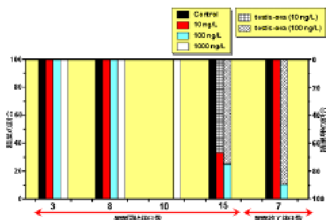
図1. 精巣卵の出現割合
