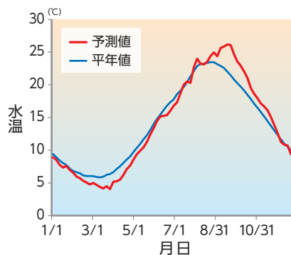
図2. 水温予測値
