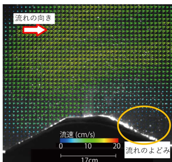
図 1 海堆周辺流れの計測実験
