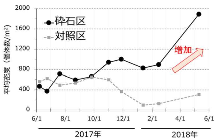
図 2 船橋市沖のアサリ密度の時間変化
