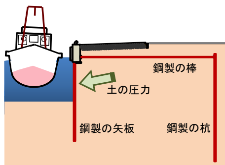
図1 矢板式係船岸
