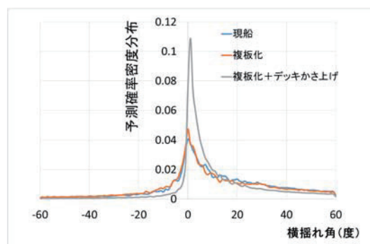
図1 横揺れ予測分布による安全性評価
