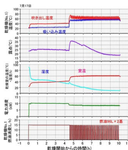
図3 コンブ乾燥施設データの一例
