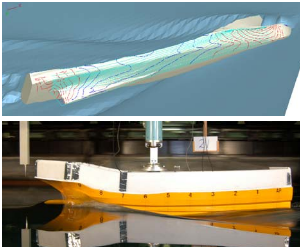
左上: 数値シミュレーションによる波紋と船体表面圧力分布(提供(有)流体テクノ)、左下: 模型実験の様子、上: 有効馬力の比較
