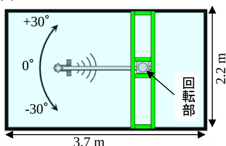
上面図
