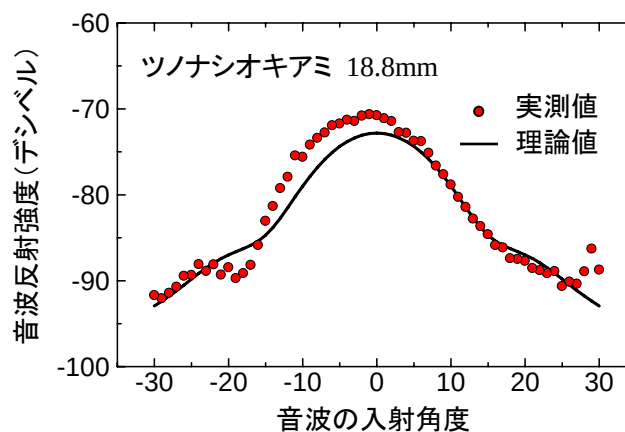
図 2. 音波反射特性の測定結果
