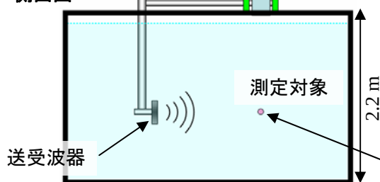
図 1. 音波反射特性の測定システム
