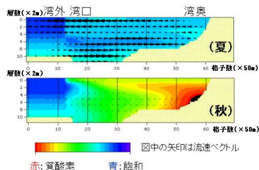
図4 溶存酸素濃度分布計算値の断面図
