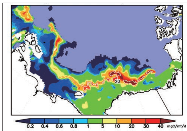
図2 モデルで予測された2017年8月14日のボーフォート海における表層の基礎生産量(mgC/m³/日; 色分け)。北極低気圧の影響を考慮した場合としない場合との基礎生産量の差が20 mgC/m³/日の海域を白色等値線で示す。紫色の領域は海水域を意味する。
