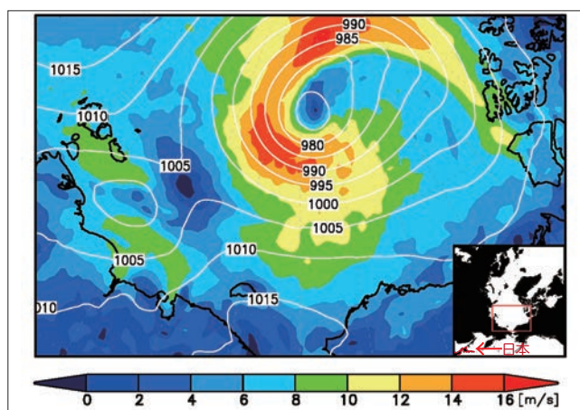
図1 2017年8月10日にボーフォート海(右下の赤枠の領域)で発達した北極低気圧の海面気圧(hPa; 等値線)と海上風速(m/s; 色分け)の日平均値。
