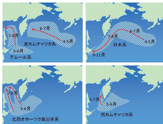
図 6. アジア系サケ成魚の回遊経路 (近藤ら 1965 を改変).
