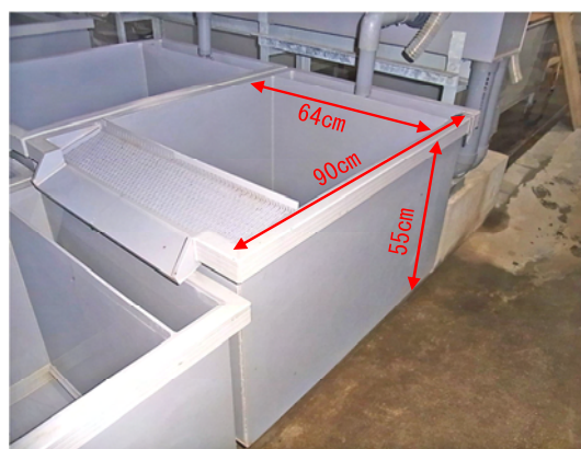
図 2. ボックス式ふ化器。
