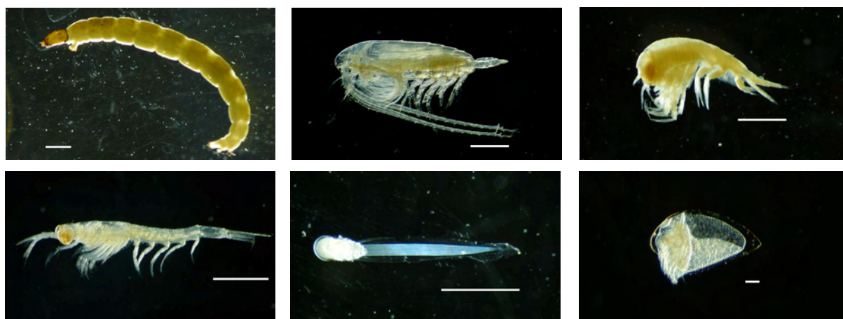
図. 河川、沿岸域におけるサケ稚魚の主な餌生物。左上：ユスリカ科の仲間。中上：カイアシ類（ Neocalanus spp.）。右上：ウミノミ類（ Themisto japonica ）。左下：オキアミ類幼生。中下：オタマボヤ類。右下：ミジンコ類。スケールバーは 1 mm、ただし左下のみは 0.1 mm。
