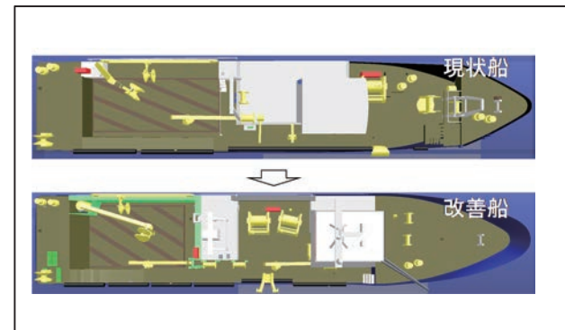
図3. 現状船（上）と改善船（下）の一般配置
