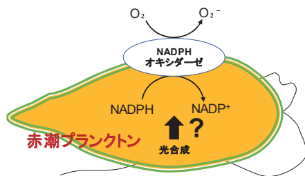
図1. シャットネラにおける O_2^- の産生機構
