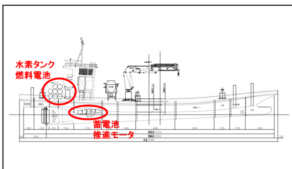
図1. 水素燃料電池マグロ養殖作業船の一般配置図
