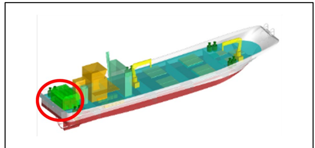
図2. コンテナ型水素燃料電池システム（○部分）による既存の養殖作業船の電動化
