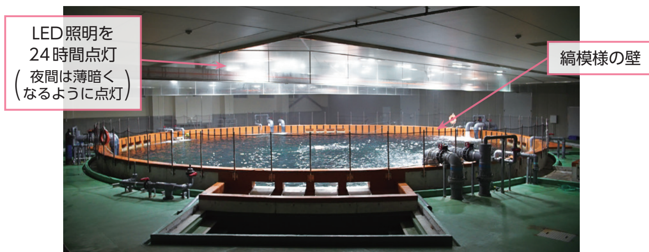
写真2 クロマグロを飼育している親魚水槽
