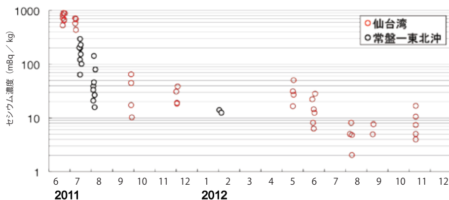
図 1 福島～仙台湾海域における海水中的放射性セシウム濃度の時間的推移 （セシウム 137 のみ表示）
