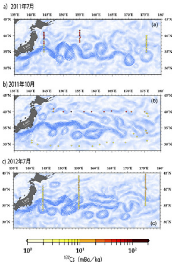
図 2 a)2011 年 7 月、b)2011 年 10 月、c)2012 年 7 月における、西部北太平洋表層の放射性セシウム濃度モニタリング結果。
