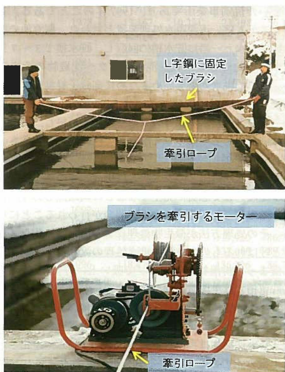
写真 1. 試作した自動清掃機のブラシと牽引モーター
