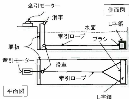
図 8. 試作した自動清掃機の仕組
