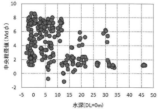
図4. 全256底泥試料の中央粒径値 (Md φ) と採泥水深との関係
