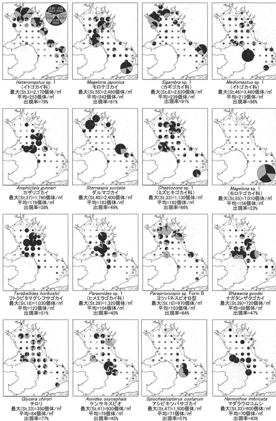
図5. 多毛類主要種の水平分布 密度 (円グラフ面積), 最大値, 平均値とも5回の調査の累積生息密度で表示, 出現率は累積生息密度が正の調査点の割合, 円グラフの黒は6月, 灰色は10月調査の生息密度を示す
