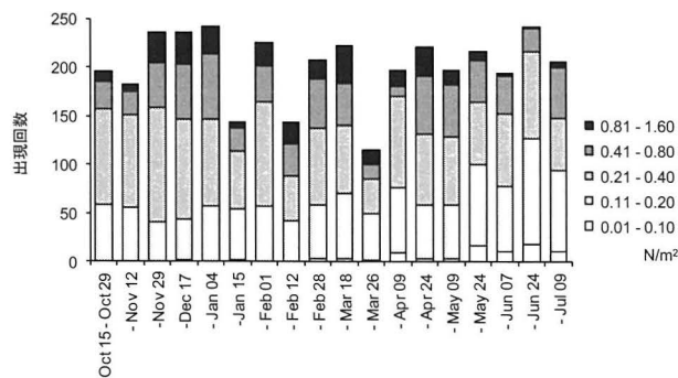
図 5. 実験 1 における底面せん断応力の出現回数 (1 パースト = 1 回) の変化
