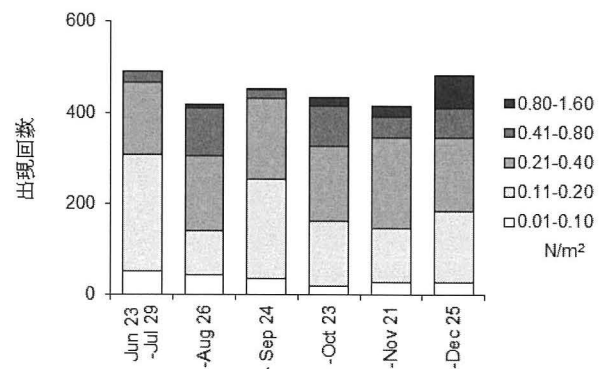
図 12. 実験 3 における底面せん断応力の出現回数の変化
