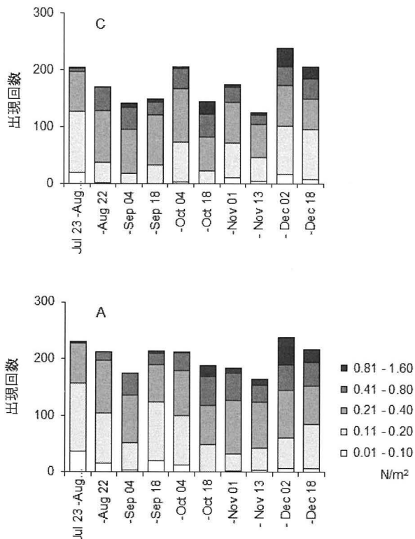
図 9. 実験 2 における底面せん断応力の出現回数の変化上, A 地点 (沖側); 下, C 地点 (岸側)
