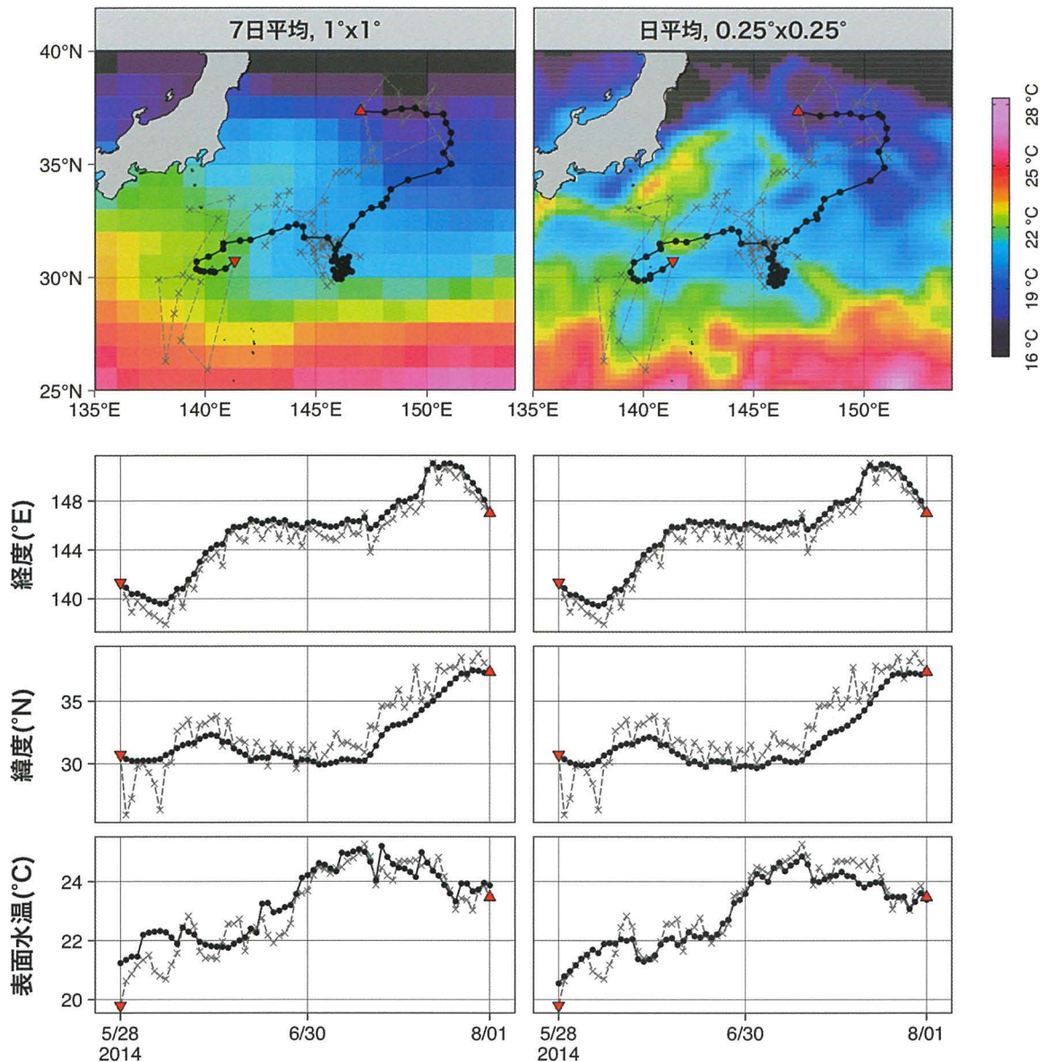
図7. 解像度の異なる海表面水温データを用いた場合のカツオ（タグ番号2601）の推定経緯度の補正例
