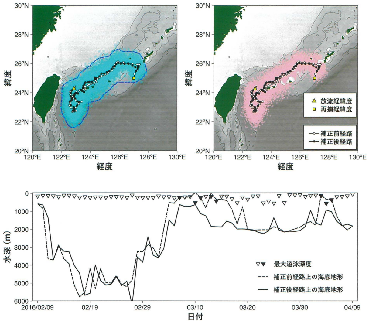
図8. 海底地形による経緯度補正の具体例（タグ番号4375）（上）海底地形による補正前（○）と補正後（●）の水平移動経路、（下）補正前経路の日最大遊泳深度（▽）と海底地形による補正前（点線）と補正後（実線）経路上の水深 この図は図2のフローの第3段階に相当する 上段の図の三角と四角の凡例はそれぞれ放流，再捕の経緯度を示す 左上図の青色の破線は海底地形による補正前経路の95%信頼区間を，薄い青色の×印はその区間内に無作為に300個発生させた経緯度を示す 右上図の薄い赤色の●印は左上図の×印のうち，海底水深がタグに記録された日最大遊泳深度よりも深い点を表す 島周りや陸棚上の●点は候補点から外れていることがわかる 下段の図の補正前経路において，日最大遊泳深度が海底地形水深よりも深い場合を▼で示す
