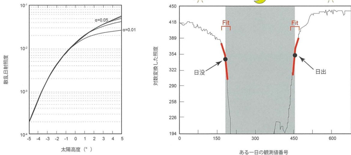
図4. Template fit法による日出・日没時刻推定の概要
