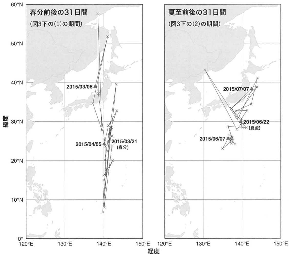
図5. カットオ（タグ番号3175）の照度に基づいて推定された経緯度の例（左）春分前後31日間，（右）夏至前後31日間 この図は図2のフローの第1段階に相当する 推定経緯度について，最初と最後の日を▲印，春分および夏至の日を●印，その他の日を×印で表す
