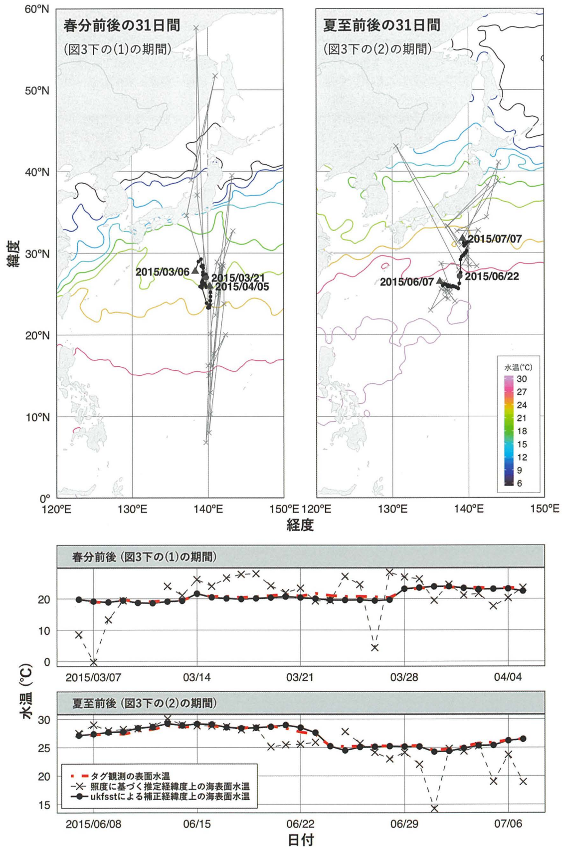
図6. カツオ（タグ番号3175）の照度に基づく推定経緯度を表面水温を考慮した状態空間モデルで補正した例（上）照度に基づく推定経緯度（×印と灰色実線）と ukfsst による補正後経緯度（●印と黒実線），（下）タグに記録された表面水温（赤色の鎖線）および春分・夏至前後における照度に基づく推定経緯度（×印と破線）と ukfsst による補正後経緯度（●印と実線）上の海表面水温 この図は図2のフローの第2段階の左の流れに相当する 春分時（上左）と夏至時（右）の人工衛星観測の海表面水温の平均値（31日間の平均）は色違いの等温線で示す
