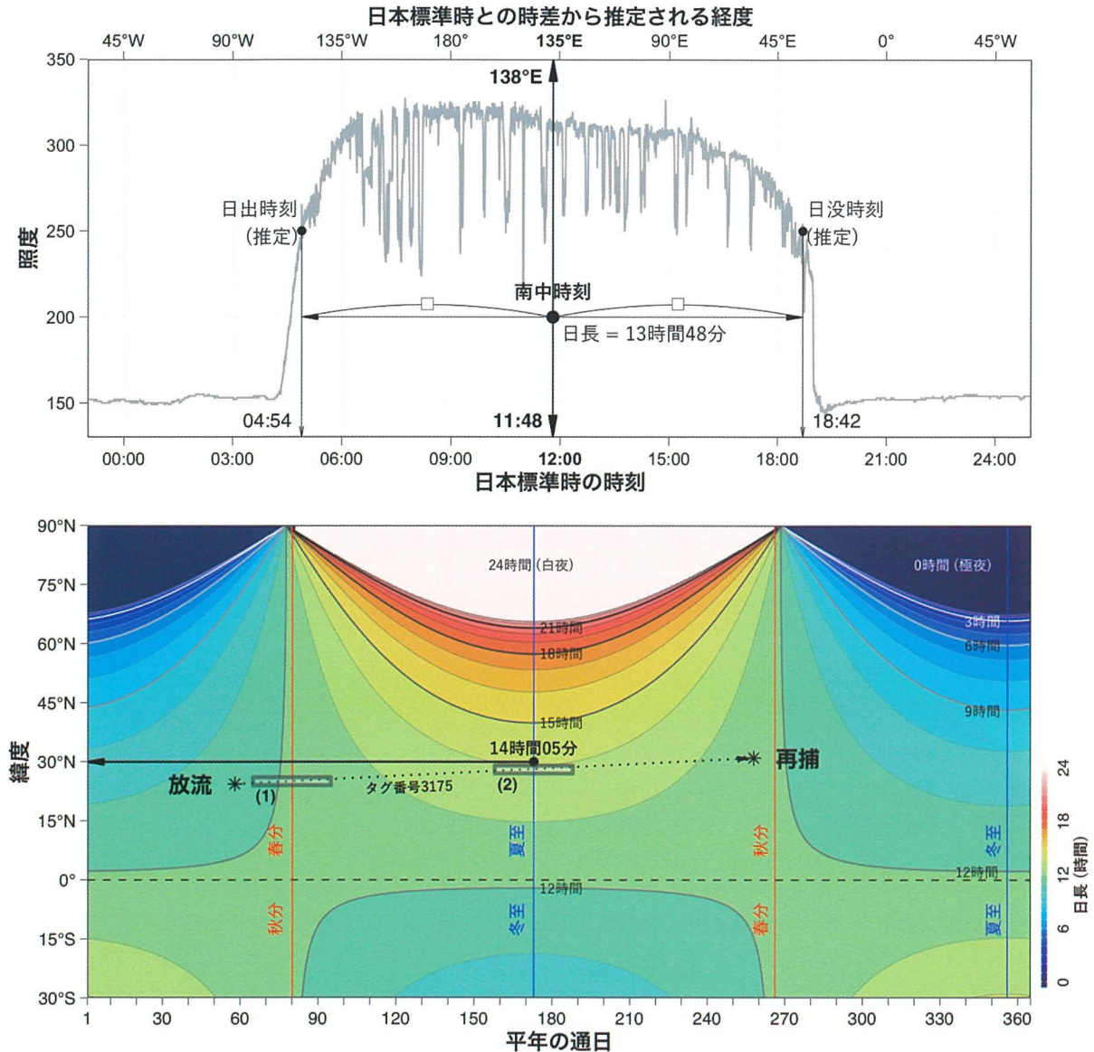
図3. タグに記録されたある一日の照度変化の例（上）と日長と緯度の関係（下） この図は図2のフローの第1段階に相当する 日出・日没時刻は照度変化から推定し、その中間時刻として南中時刻（11:48）、また、日長（13時間48分）を計算する 下図の赤線は春分・秋分を、青線は夏至・冬至を示す 照度による経緯度補正に使用した個体（タグ番号3175）の放流から再捕までの期間を点線で結んだ (1), (2) で示した期間のデータは図5、図6で照度による経緯度推定結果を例示する
