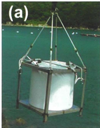
写真1. (a) キャンバスシート製バケツ (直径80cm, 深さ80cm, 容量400L), (b) ターポリンシート製担架 (長さ80cm, 深さ35cm)
