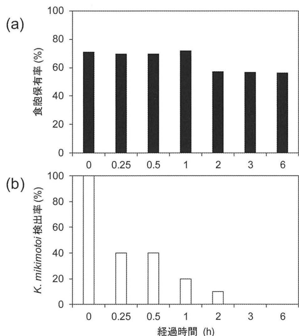
図2. Karenia mikimotoi を摂食させた Noctiluca scintillans ( n > 50 )の食胞保有率 (a) および食胞が認められた N. scintillans ( n = 10 )のLAMP法による K. mikimotoi 検出率 (b)、摂食させた後、ろ過海水に移してから0～6時間経過した時点で固定し、分析した
