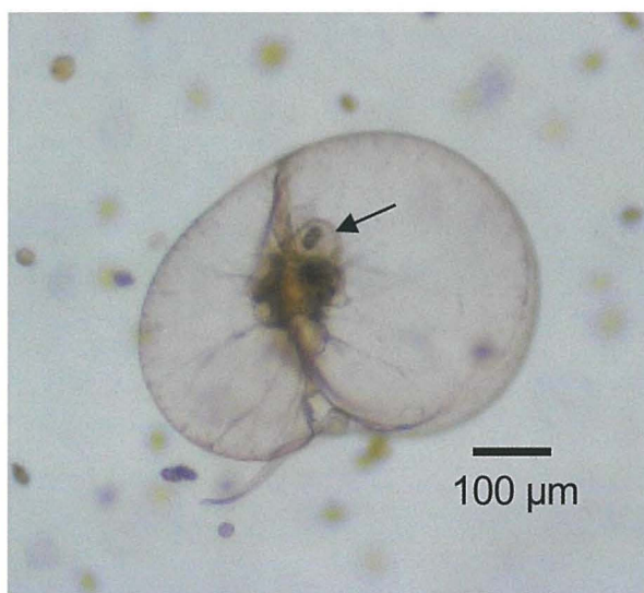
図1. Karenia mikimotoi を摂食した Noctiluca scintillans 、矢印は食胞を示す
