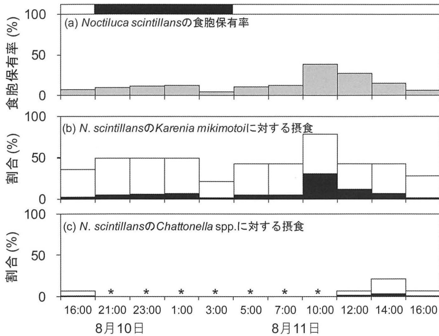
図4. 2015年8月10～11日の英虞湾における Noctiluca scintillans の食胞保有率 (a), 食胞を保有している N. scintillans (各時刻において n = 14 ) が Karenia mikimotoi を摂食していた割合 (白) および全体のうち K. mikimotoi を摂食していた割合 (黒) (b), 食胞を保有している N. scintillans (各時刻において n = 14 ) が Chattonella spp. を摂食していた割合 (白) および全体のうち Chattonella spp. を摂食していた割合 (黒) (c) *は検出されず。全体のうち K. mikimotoi あるいは Chattonella spp. を摂食していた割合 (黒) は N. scintillans の食胞保有率 (a) に N. scintillans ( n = 14 ) が K. mikimotoi あるいは Chattonella spp. を摂食していた割合 (b, cの白) を乗じて算出した 上部の白色部分は昼間, 黒色部分は夜間を示す
