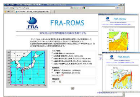
新しい海況予測システム「FRA-ROMS」
