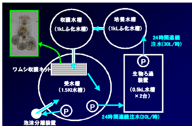
図2 閉鎖循環式フムシ連続培養システムの模式図。矢印は海水の流れを示す。
