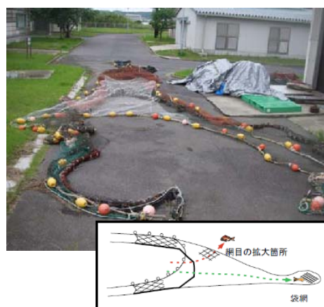
タイ類の資源を有効利用する底びき網
