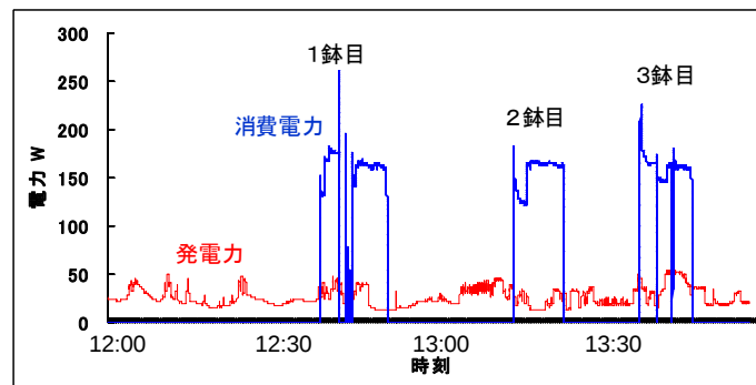
立て縄操業時の太陽光パネル発電力と消費電力
