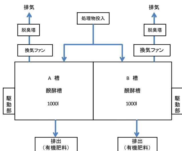
設備図
