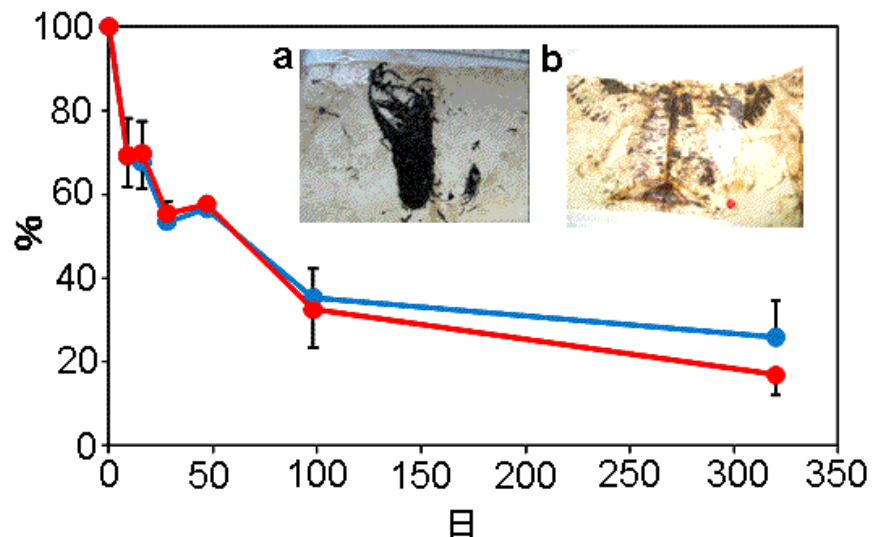
図2 網袋に封入し、海底に設置したノコギリモクの未分解藻体の重量（●）および炭素量（●）の経時変化（初期量に対する相対値）。写真は1ヵ月後（a）および320日後（b）の未分解物を示している。
