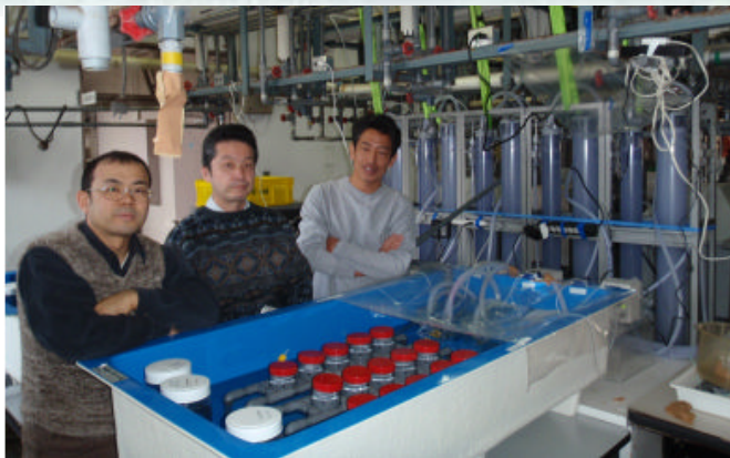
図1 二酸化炭素濃度調整装置（右：メインコントローラー、左奥：二酸化炭素ガスを海水に溶け込ませる吸収塔大小）と、様々な二酸化炭素濃度で調整した海水でエゾアワビ初期幼生を飼育する実験装置（左手前）。
