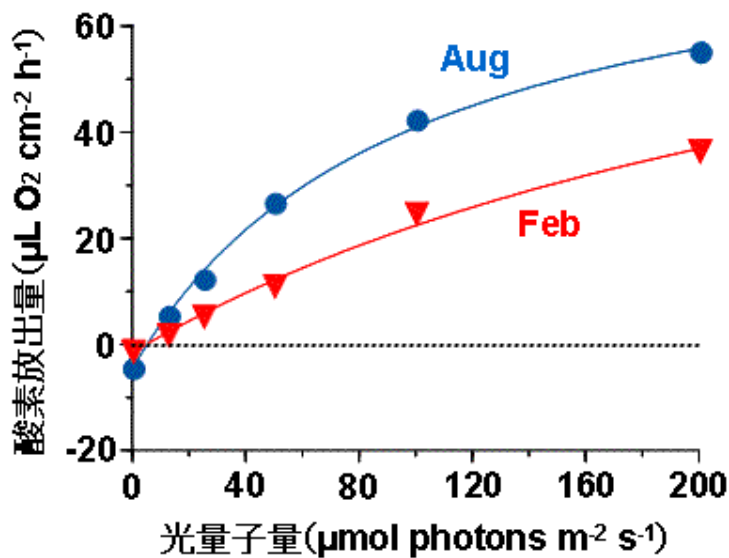
図1 最高水温時（27℃、8月）および最低水温時（10℃、2月）に採集したノコギリモクの光合成速度（酸素放出量で表記）と光量子量との関係。実線は実測値に半飽和型のモデル式をあてはめた時の推定値を示している。
