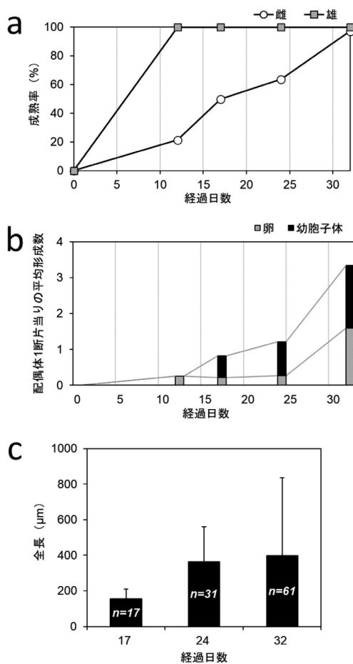
図2. アラフリー配偶体の成熟・受精確認試験の結果
