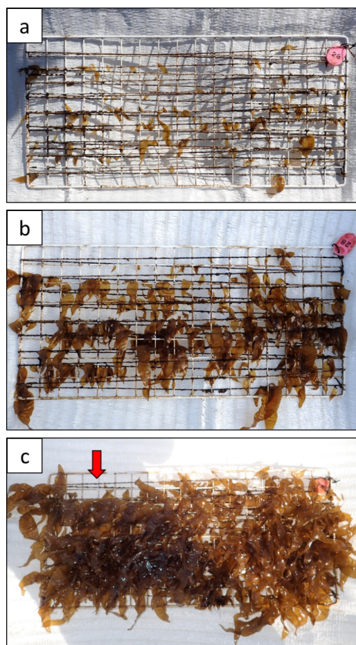
写真 6. 育苗期間におけるアラメ種苗の状態
