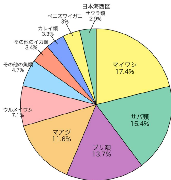
図2.3.2b 2019年の海面漁業生産統計にもとづく日本海西区の漁獲物の種組成
