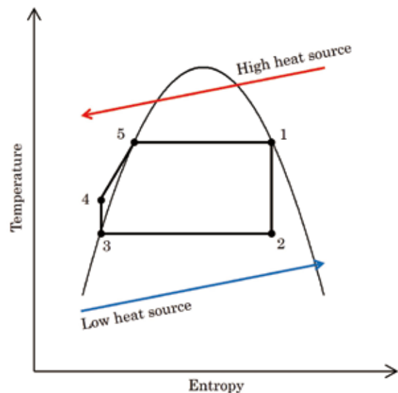
Fig. 2. T - s diagram.
